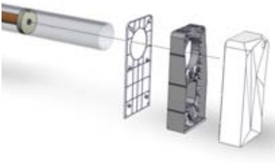
Eje de aluminio integrado en el pie Para un acabado estético pero también para protegerlo de las inclemencias climáticas.
